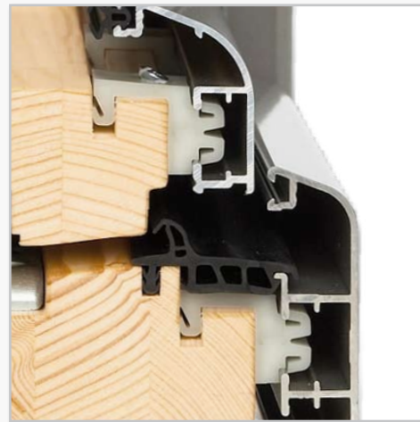
Profilgeometrie
